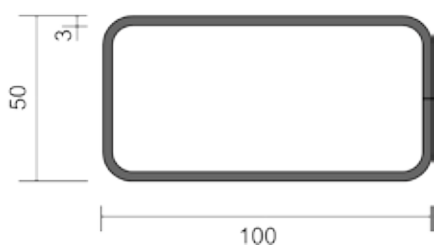
VS 571335 - Stålrör 100x50 mm
