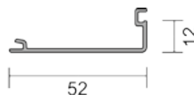
VP 45.400 - Täckprofil till 45.100
