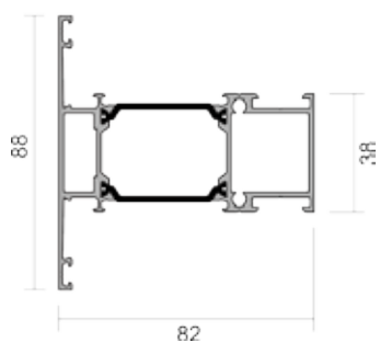
72.5838 - Spröjsprofil Fönster
