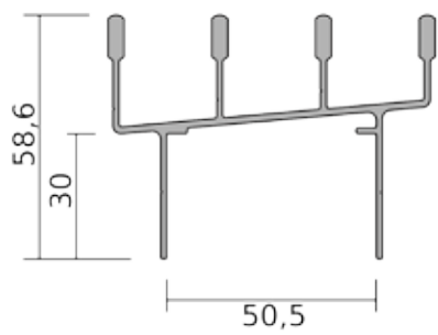
VP 60-4B - Rällsprofil 4-spår U
