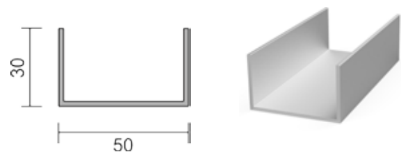
SP U5030 U profil 50 x 30 x 2 mm
