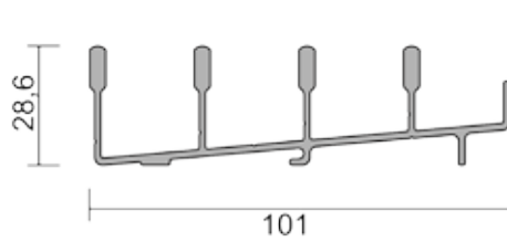
VP 60-4DR - Rällsprofil med drän, ränna 4-spår
