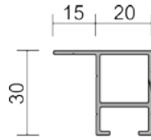
VP 65 - Profil fasta partier
