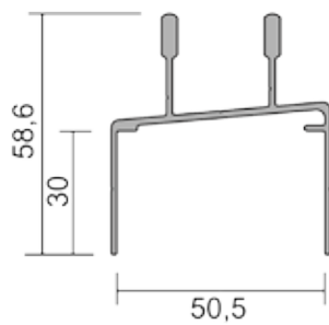
VP 60-2B - Rällsprofil 2-spår U
