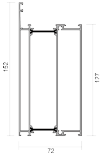
72.3127 - Karmprofil
