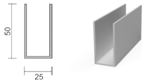
SP U2550 U profil 25 x 50 x 2 mm
